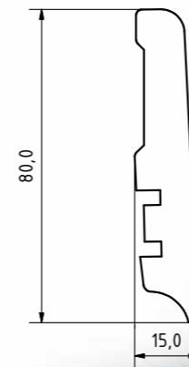
Plinthe F80 : 15x80x2500 mm Skirting F80 Rodapié F80
