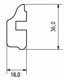
Moulure mur/plafond : 16x36x2500 mm Molding wall / ceiling Moldura pared / techo
